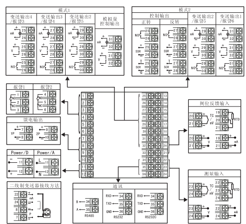
NHR-7330(R)系列仪表接线图
