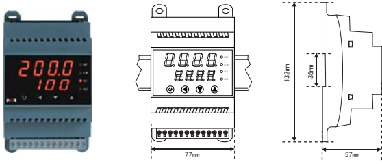
外形尺寸: 宽*高*深: 77×132×57mm
