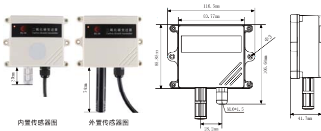
外形尺寸：宽*高*深：116.5×85.85×41.7mm
