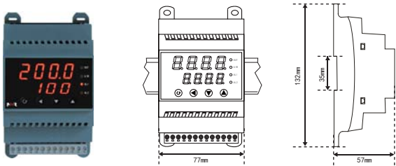
外形尺寸: 宽*高*深: 77×132×57mm
