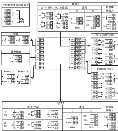
规格尺寸为F型接线图
