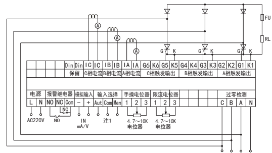
7、三相半控整流KZ3
