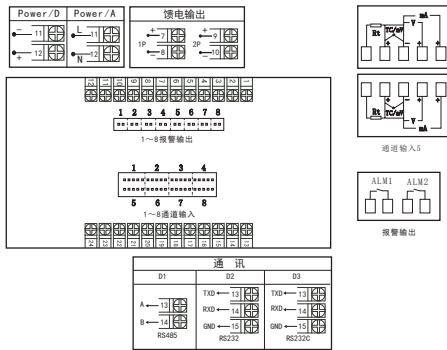
C型分别变送接线图
