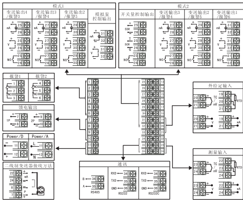
NHR-7320(R)系列仪表接线图
