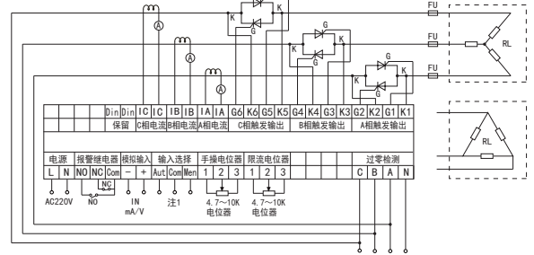
4、三相全控KP3（单向可控硅反并联，△形接法或Y形接法星点不接N）
