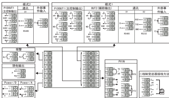
规格尺寸为F型接线图
