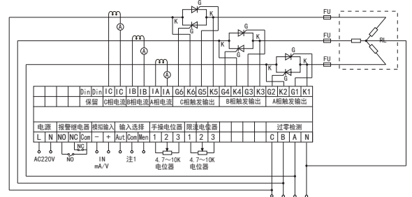
8、三相KP4（单向可控硅反并联，Y形接法星点接N）
