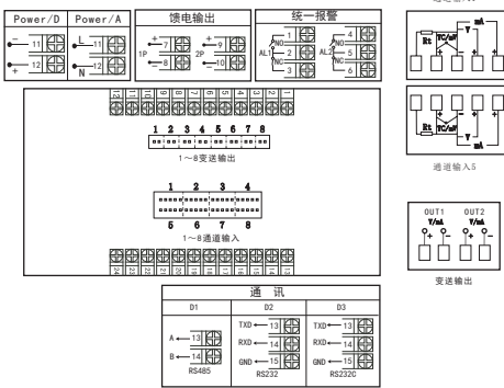
C型分别变送接线图
