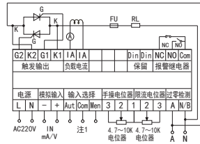
3、单相控制KZ1（半控桥式整流）
