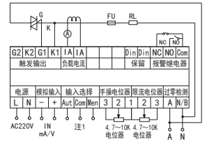
2、单相控制KS1（双向可控硅）
