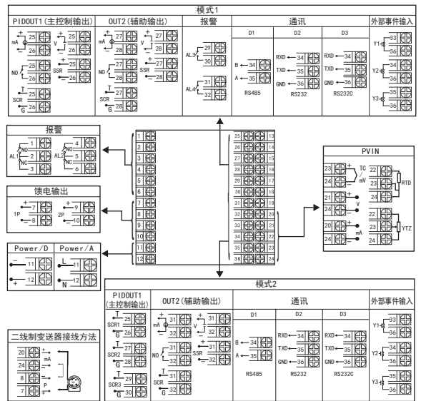
规格尺寸为A、B、C、D、E、K、L、M型接线图 注：横竖式仪表后背接线端子方向不一样，见示意图1
