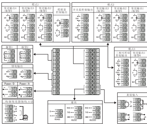
NHR-7320(R)系列仪表接线图
