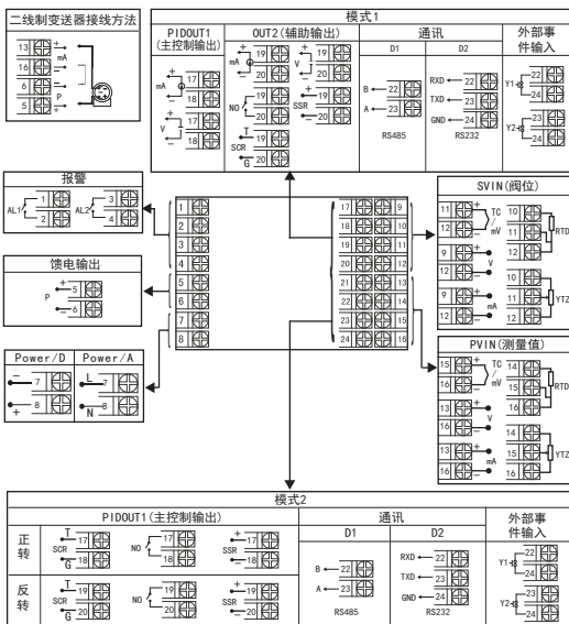
规格尺寸为F型接线图
