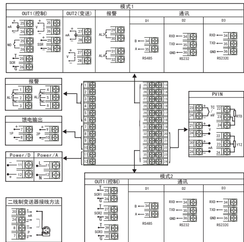
规格尺寸为A、B、C型接线图 注：横竖式仪表后盖接线端子方向不一样，见示意图1
