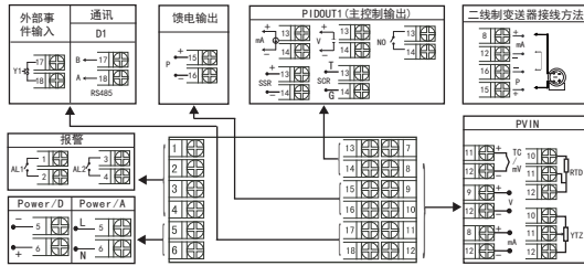
规格尺寸为H型接线图
