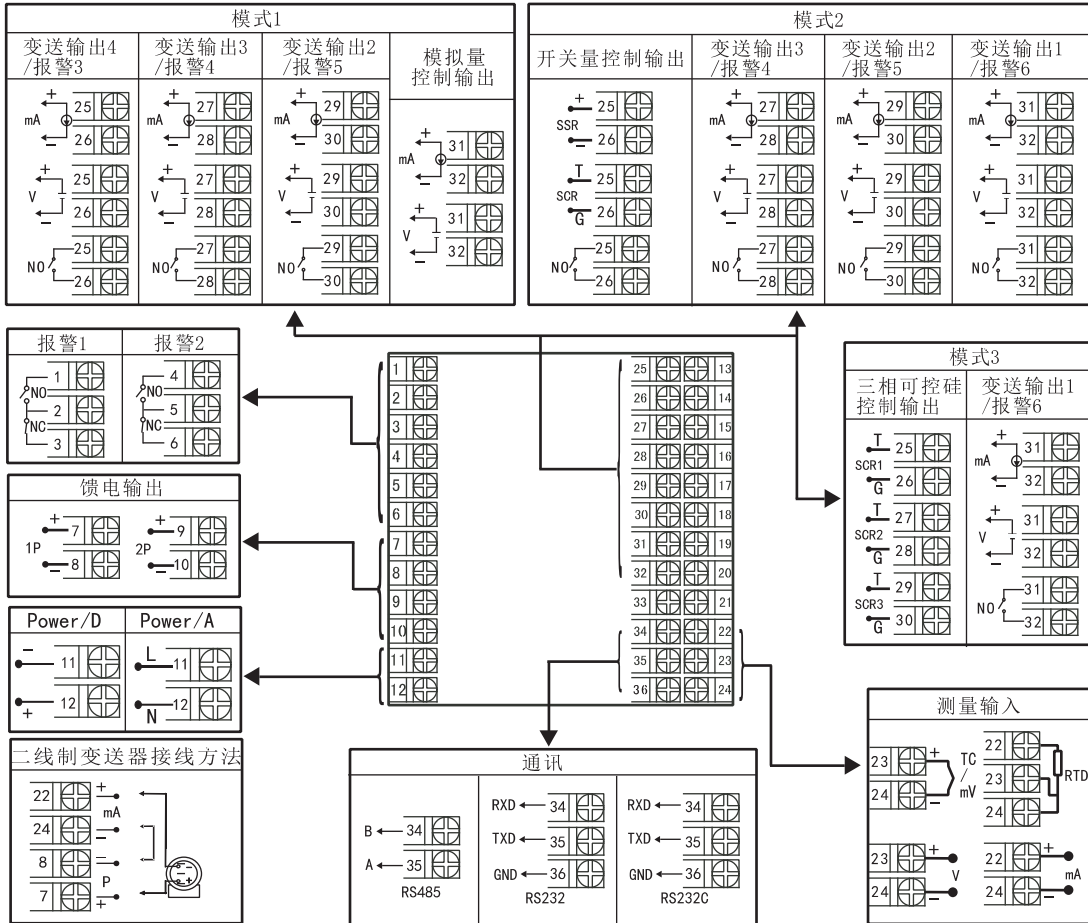
NHR-7310/7340系列仪表接线图
