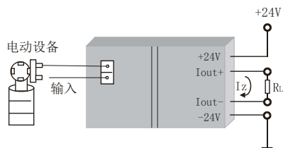
接线图一
