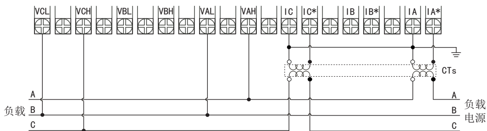
1-3、三相综合电量采用无CT、PT接入接线图（适用于3P3L）
