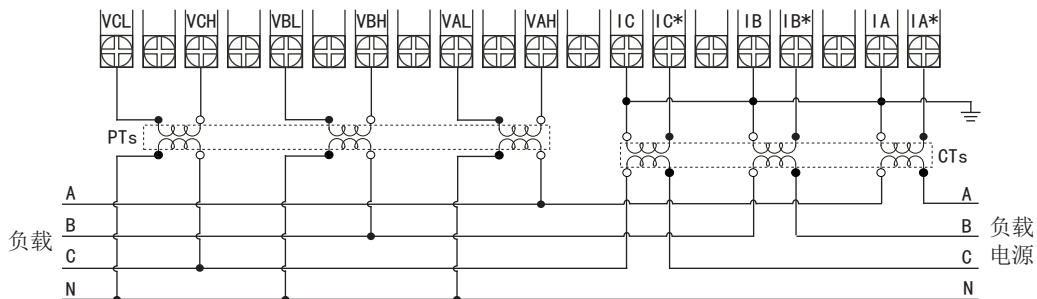
2-2、三相综合电量采用CT、PT接入接线图（适用于3P4L）
