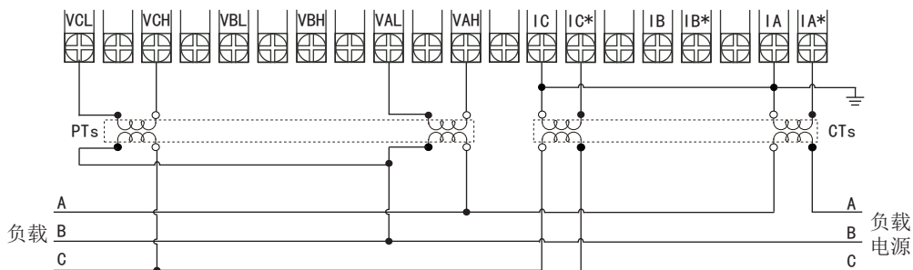
1-2、三相综合电量采用CT、PT接入接线图（适用于3P3L）
